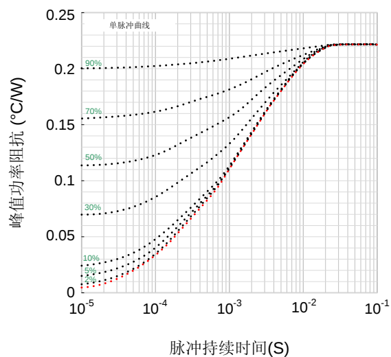
图14. IGBT瞬态热阻抗
