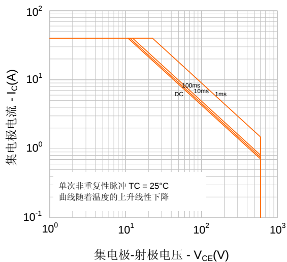
图13. SOA特性
