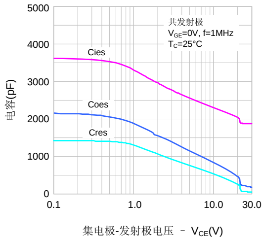
图7. 电容特性
