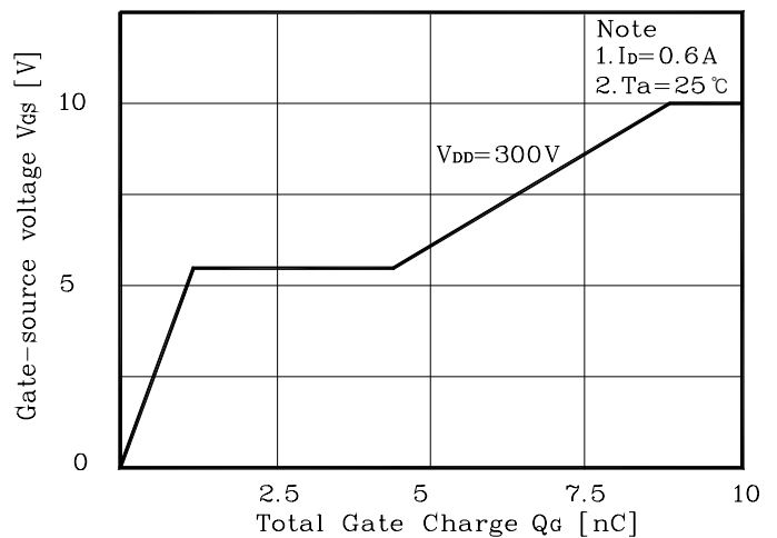
Fig. 6 V_{GS} - Q_G
